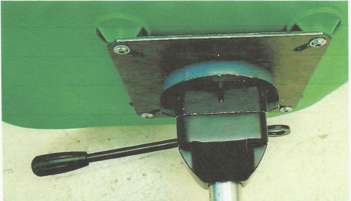
„3D-Sitzlagerung mit Härteeinstellung“ mit beispielhaft montierter Sitzfläche und Drehkreuz (linker Hebel: Höhenverstellung Stuhl; rechter Hebel: Härtegradeinstellung/ Neigungseinstellung)
